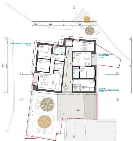
SOTTOTETTO 1:200
