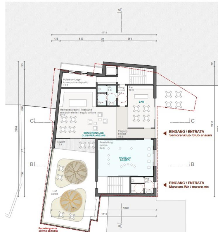
ERDGESCHOSS 1:200
