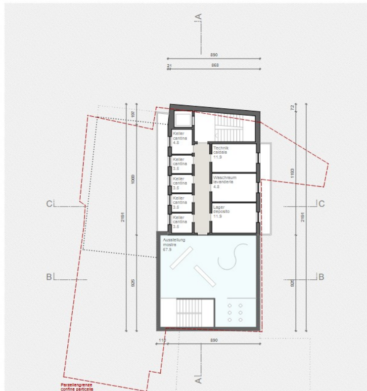
UNTERGESCHOSS 1:200
